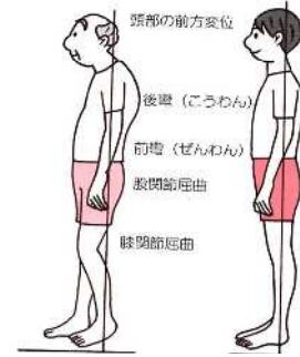
図1 老化による姿勢の変化
